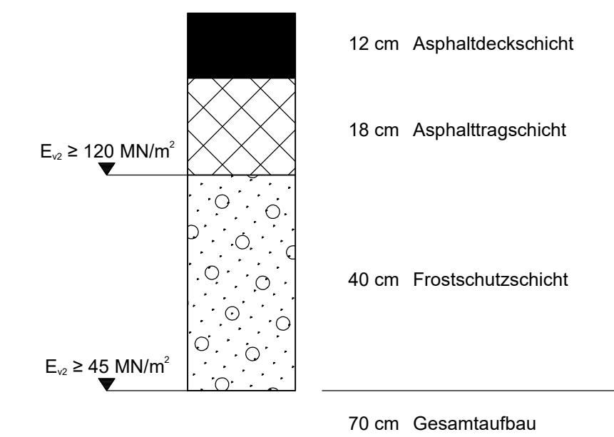
Fahrbahnaufbau nach RStO 12 Tafel 1: Belastungsklasse 32; Zeile 1
