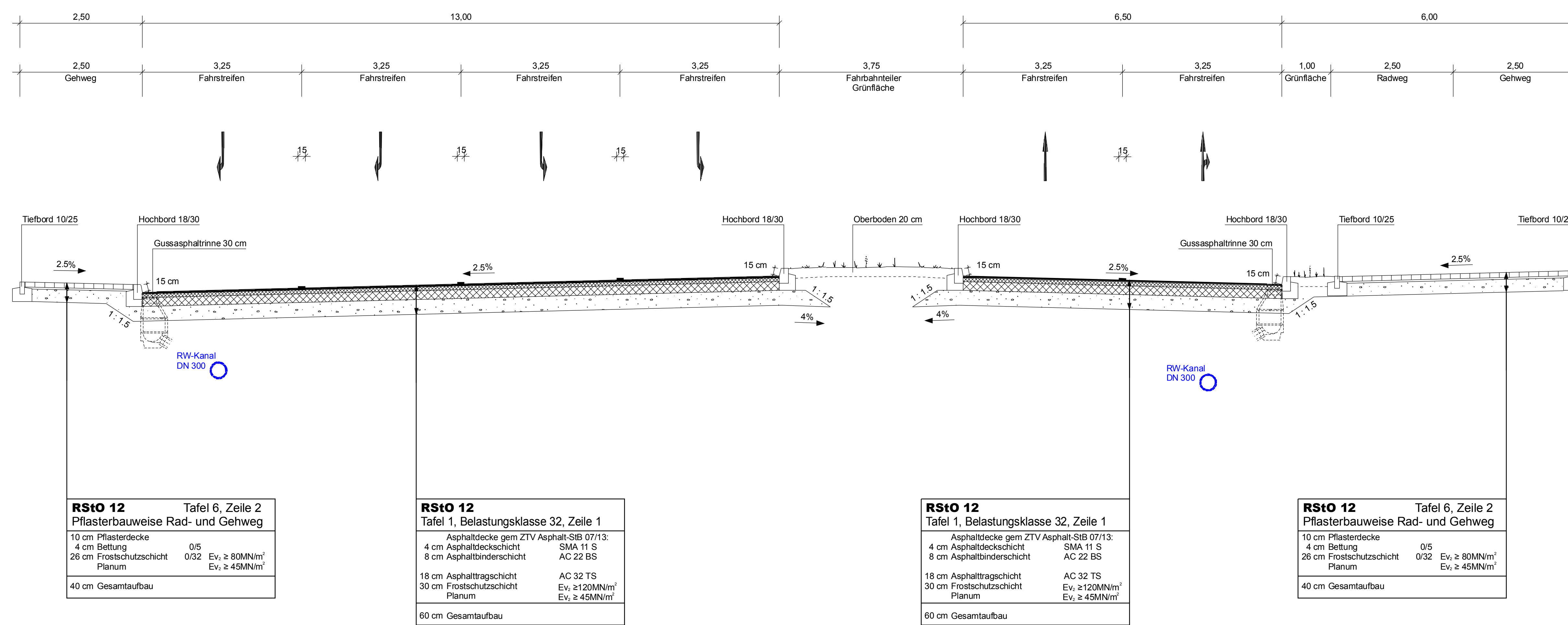
Regelquerschnitt 09 Bürgermeister-Grünzweig-Straße
