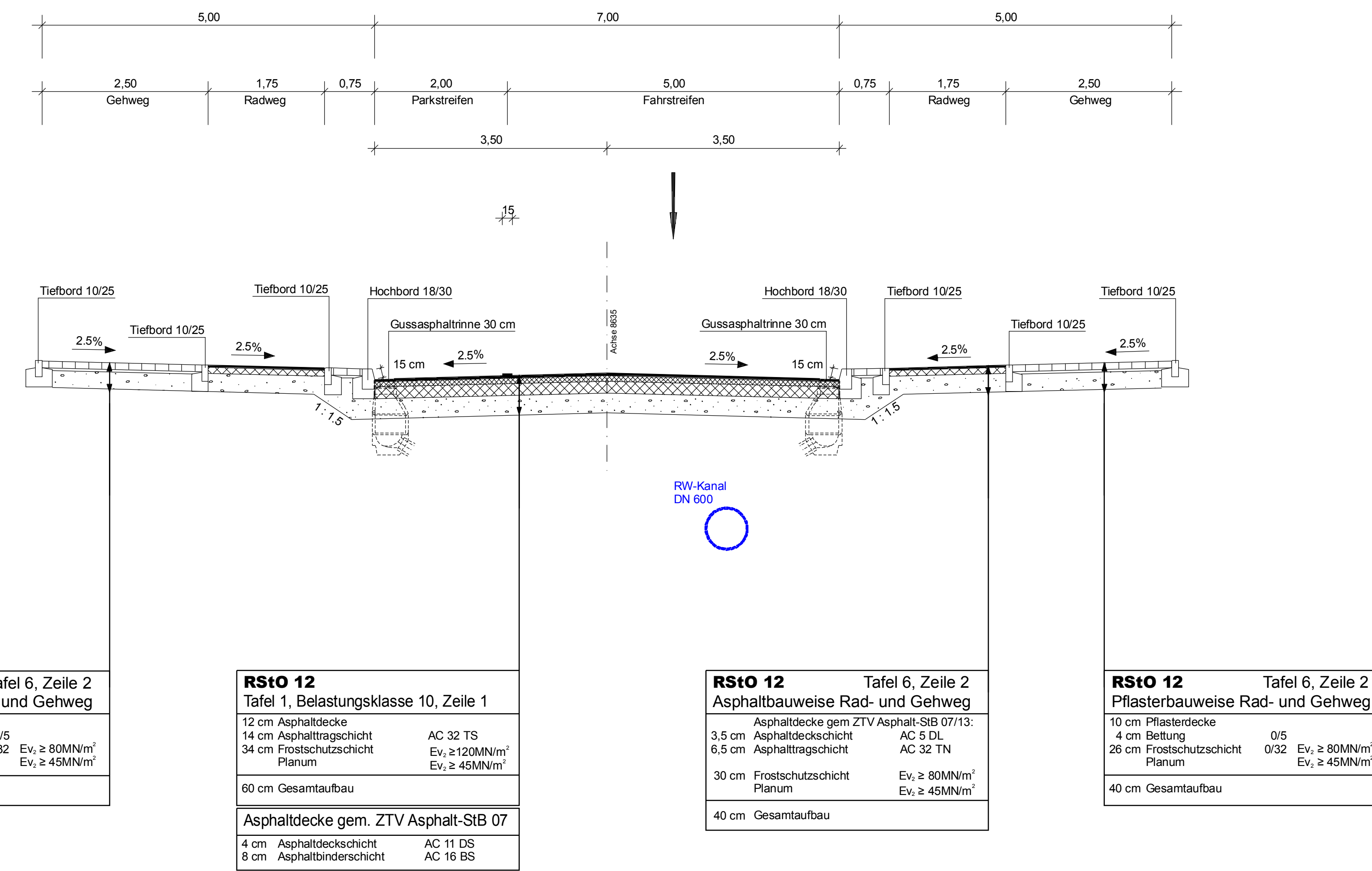
Regelquerschnitt 08 Planstraße
