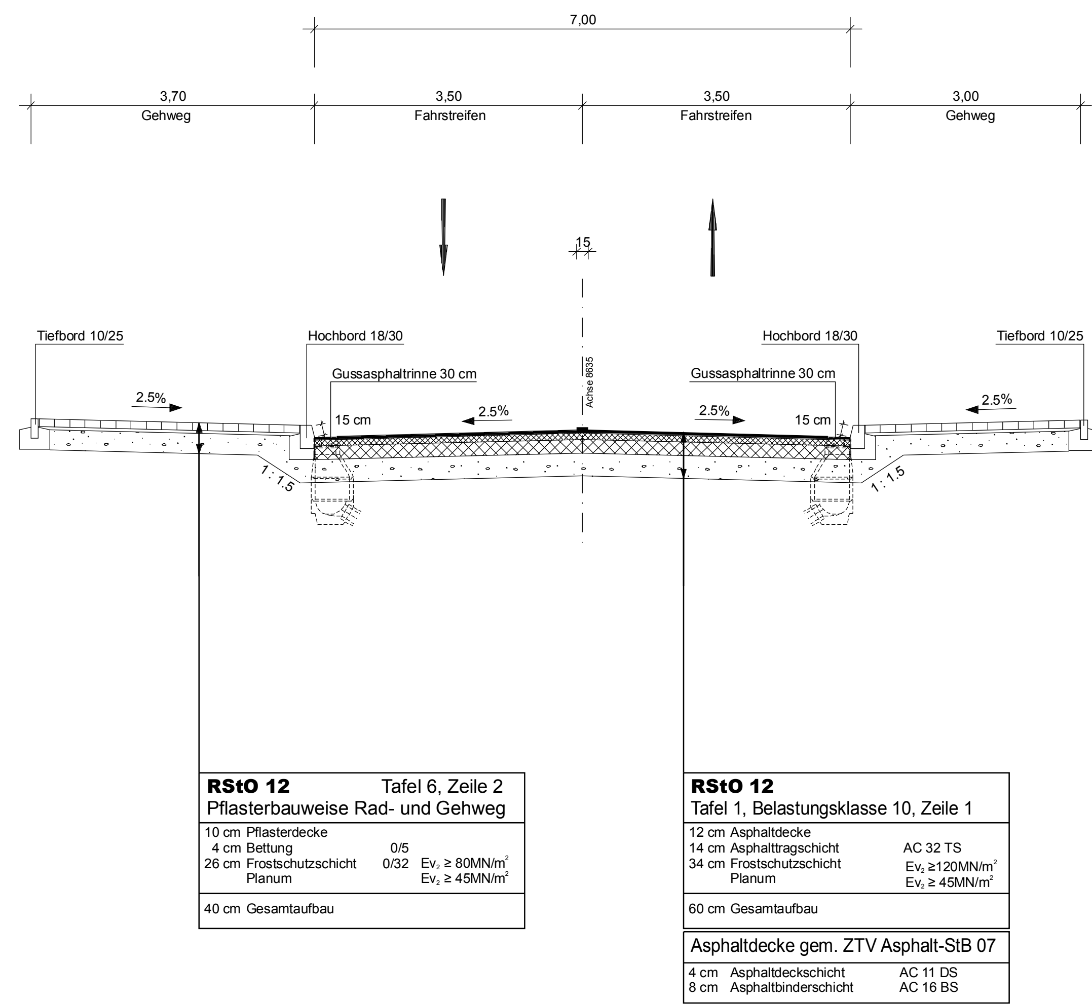
Regelquerschnitt 07 Jägerstraße
