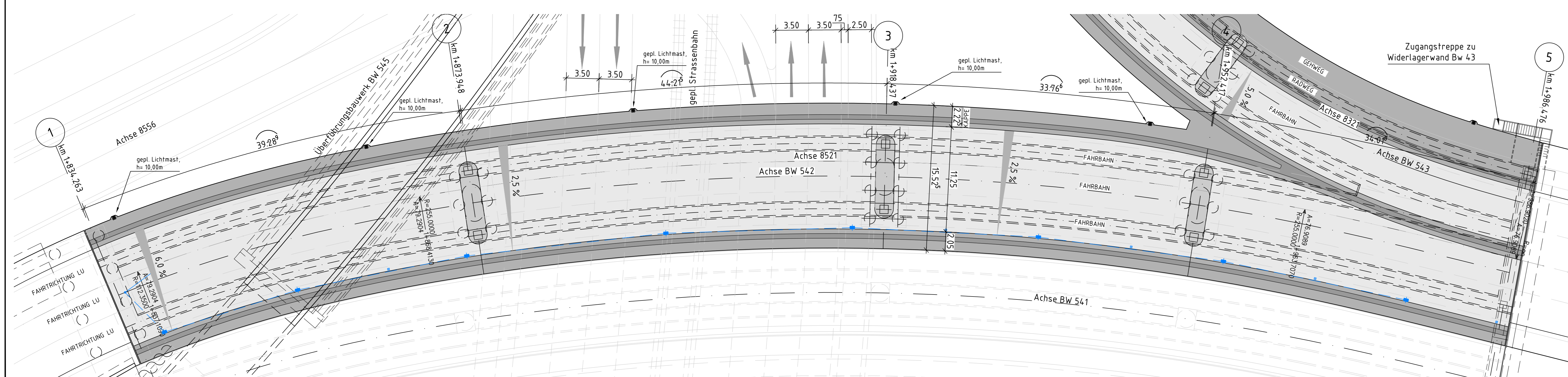
Grundriss Überbau M 1:200
