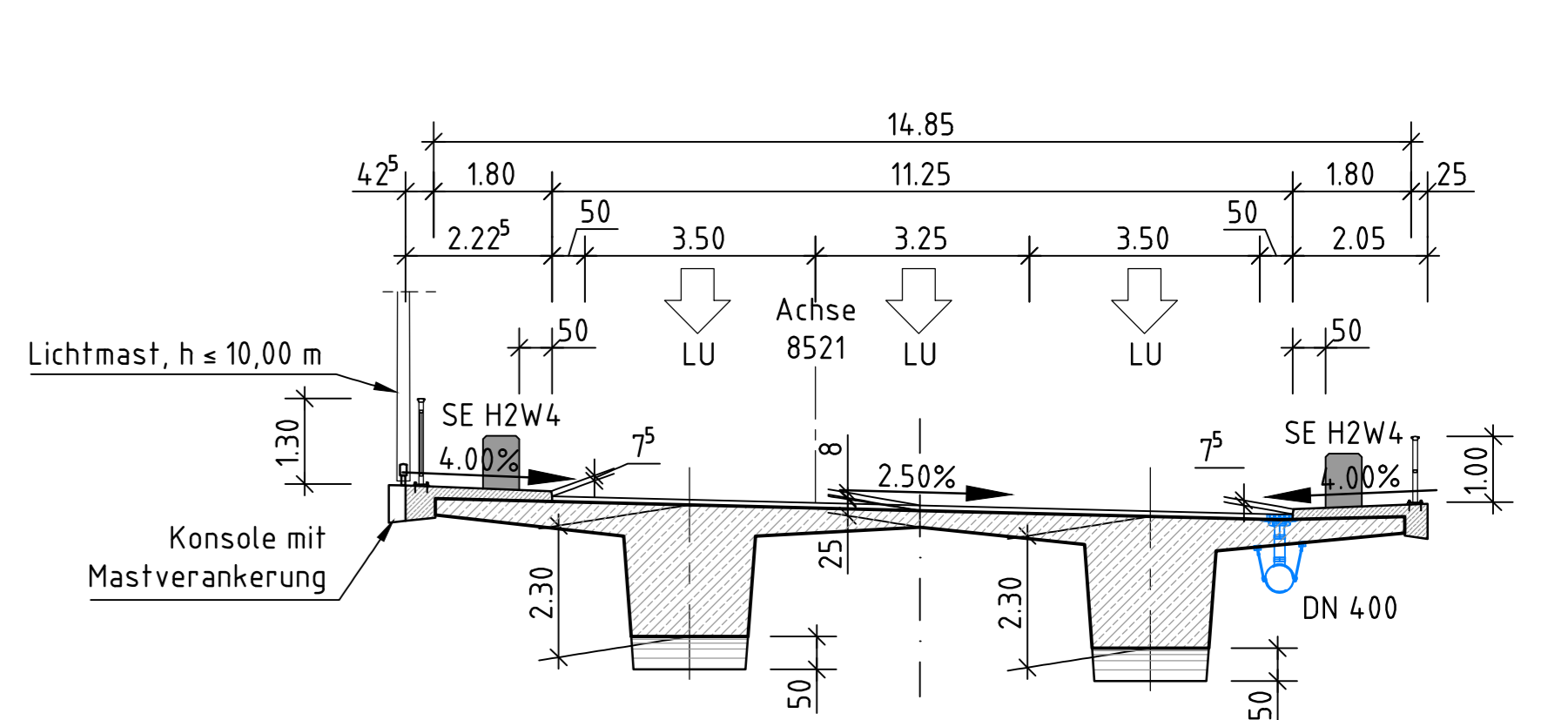
Regelquerschnitt in Feldmitte M 1:100
