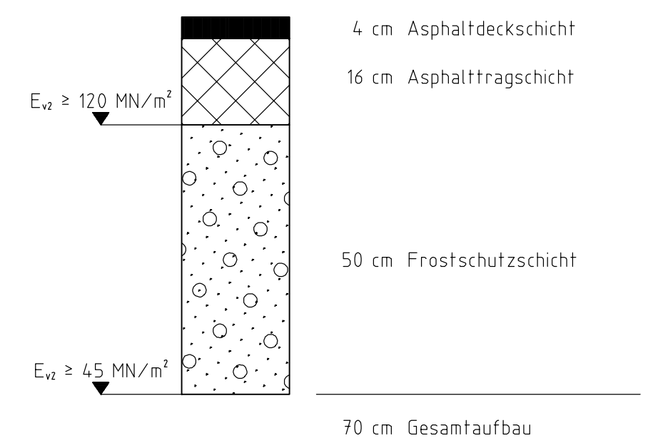
Fahrbahnaufbau nach RStO 12 Tafel 1: Belastungsklasse 1,8; Zeile 1
