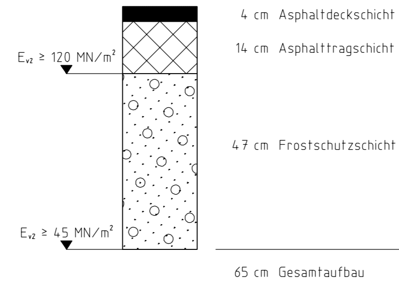
Fahrbahnaufbau nach RStO 12 Tafel 1: Belastungsklasse 1,0; Zeile 1
